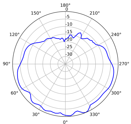
5GHz (Vertical)
